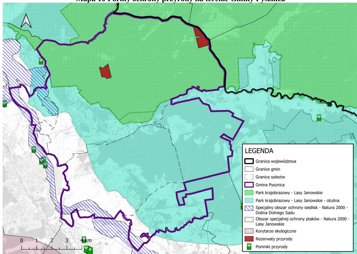
Mapa 10 Formy ochrony przyrody na terenie Gminy Pysznica
