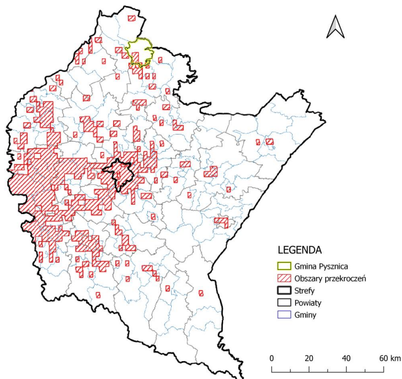
Mapa 11 Zasięg obszarów przekroczeń średniorocznego poziomu docelowego B(a)P określonego ze względu na ochronę zdrowia w województwie podkarpackim w 2021 r.
