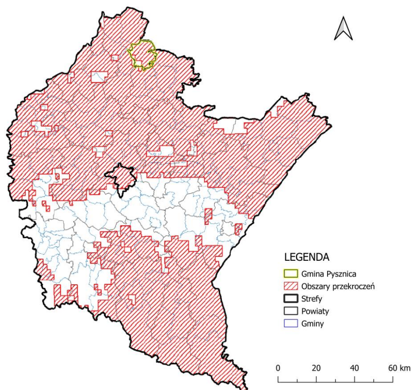
Mapa 12 Zasięg obszarów przekroczeń poziomu celu długoterminowego ozonu dla 8-godz. Stężenia O_3 ze względu na ochronę zdrowia w województwie podkarpackim w 2020 r.
