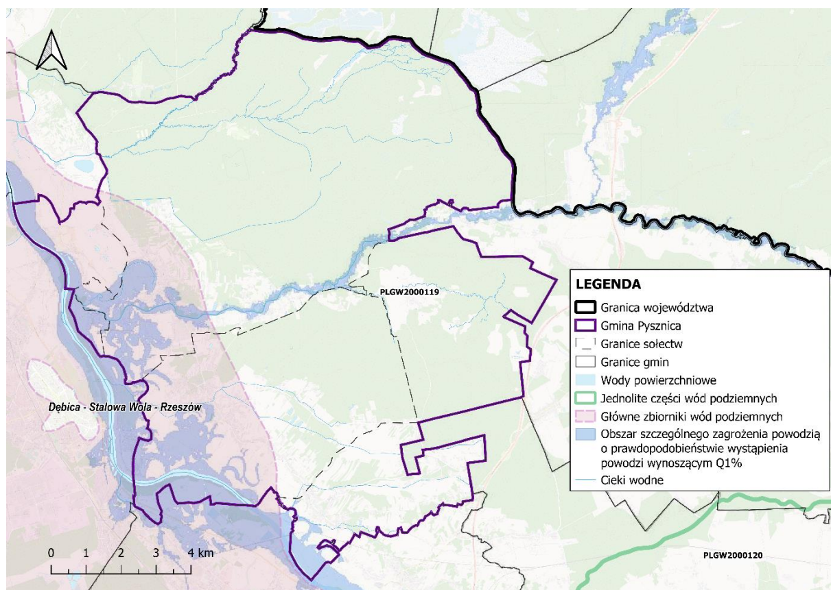
Mapa 13 Obszar zagrożenia powodziowego na terenie Gminy Pysznica
