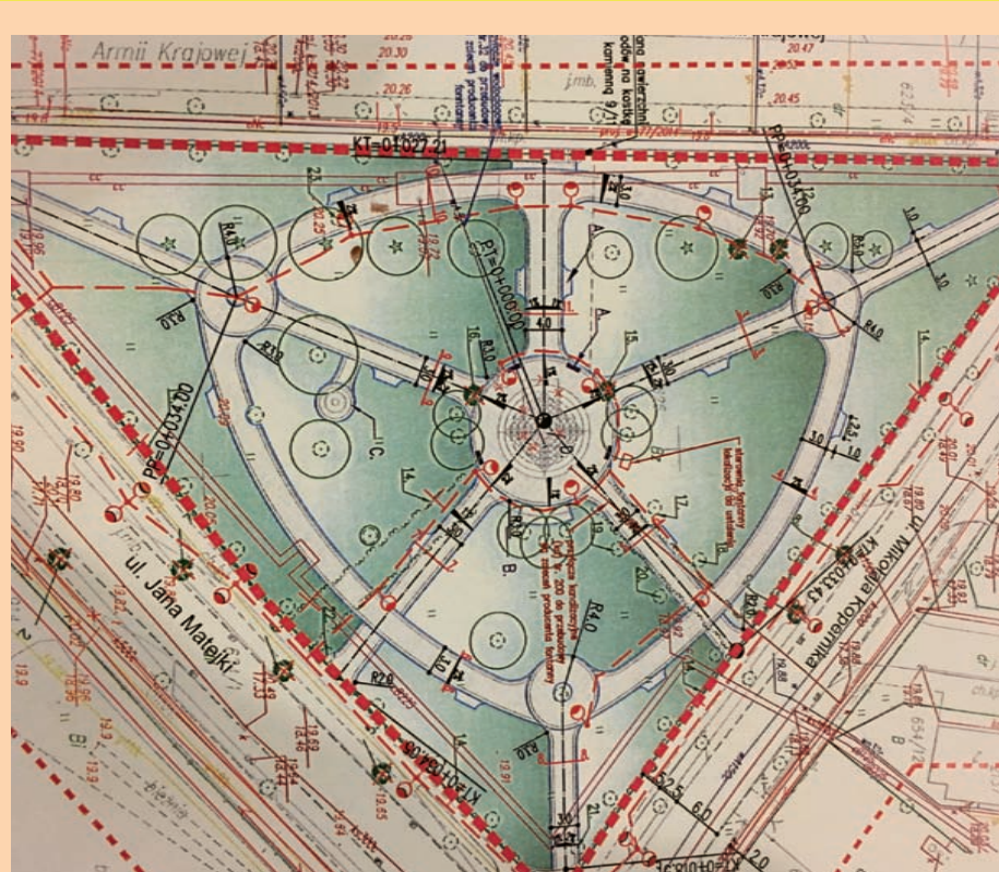
Projekt zagospodarowania skweru przy ul. Armii Krajowej
