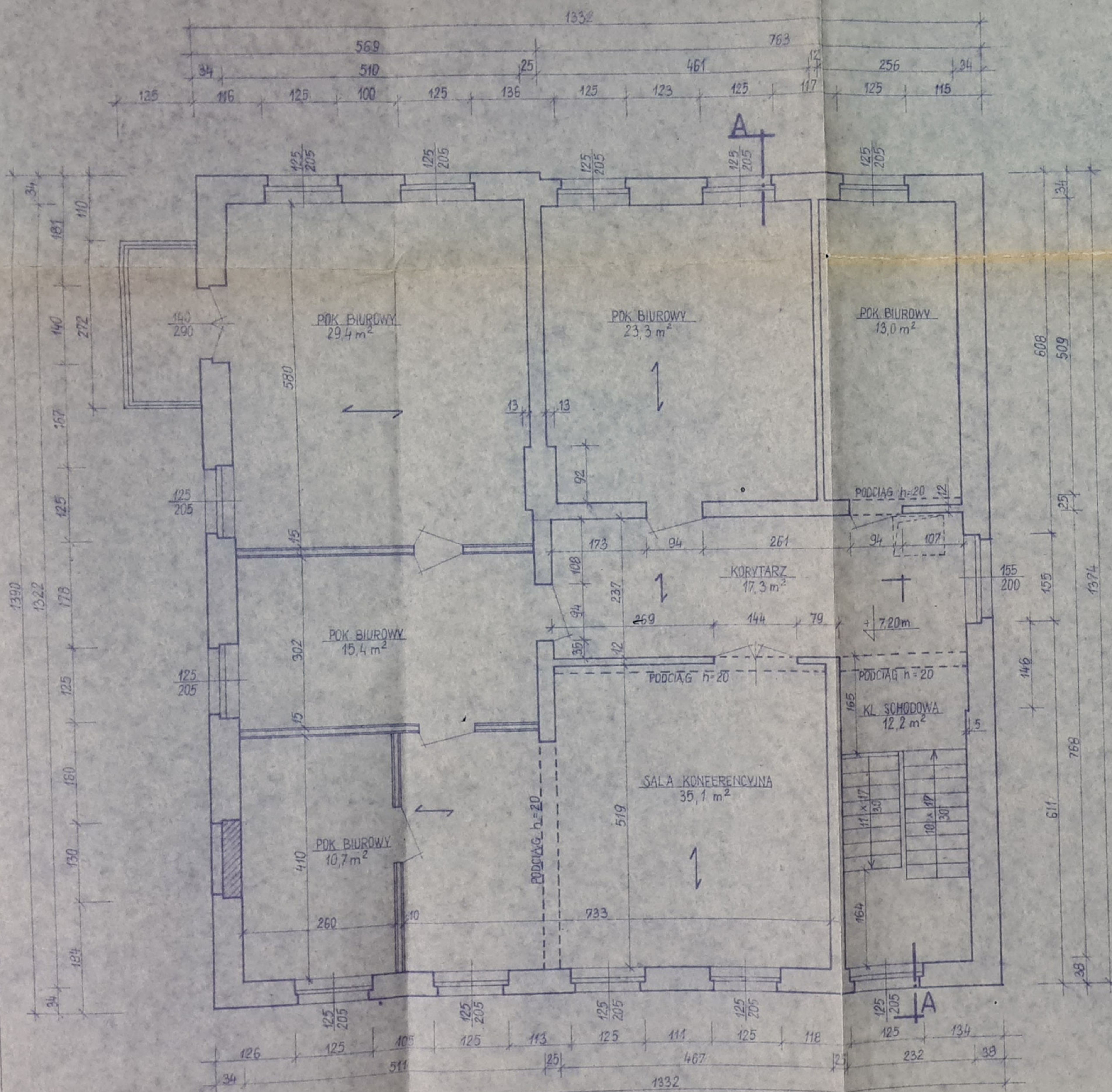
RZUT II PIĘTRA 1:50
