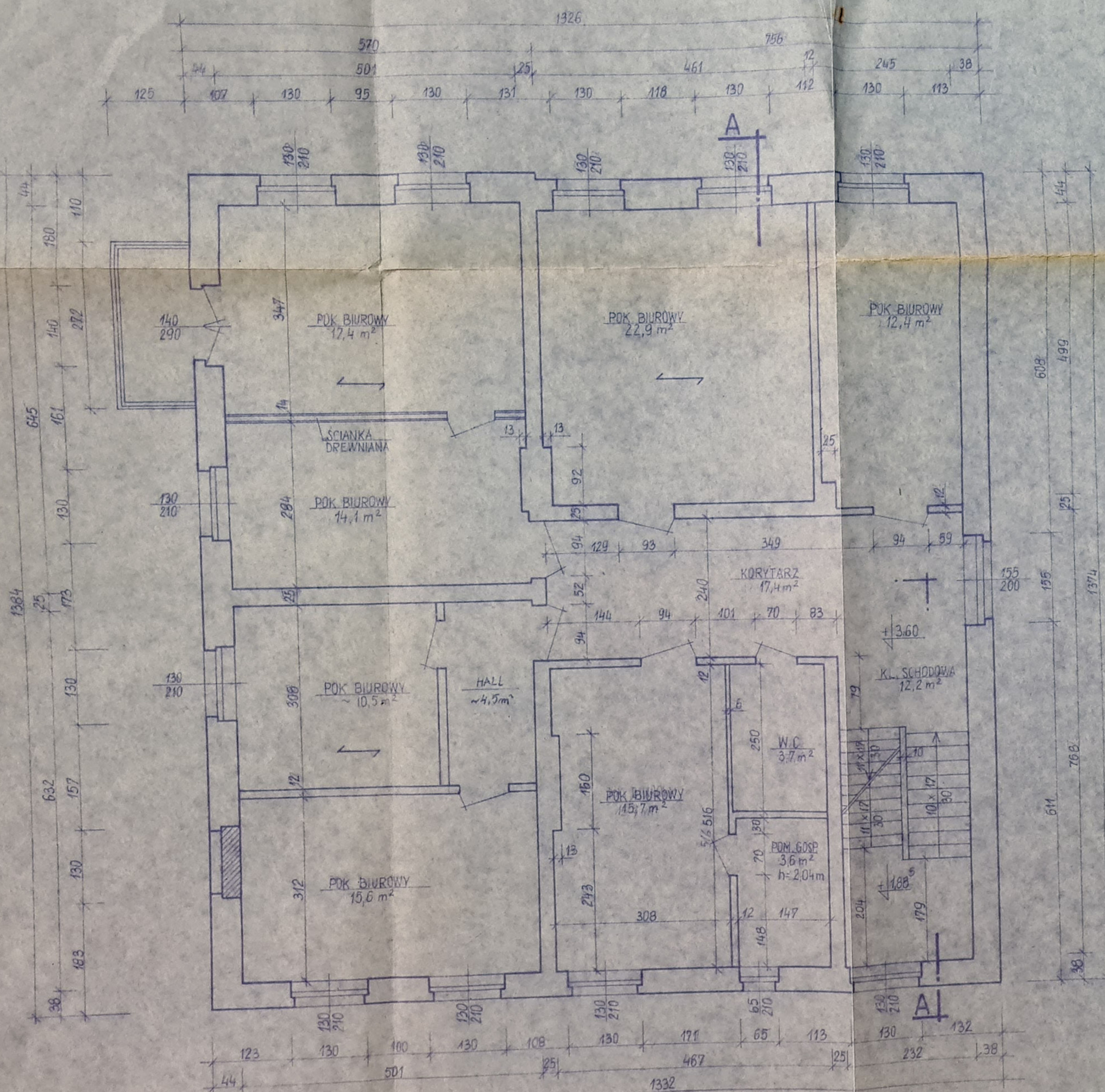
RZUT I PIĘTRA 1:50
