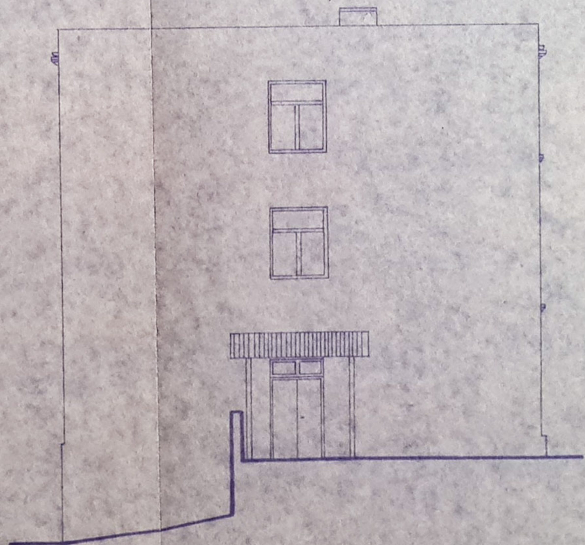
ELEWACJA WSCHODNIA
