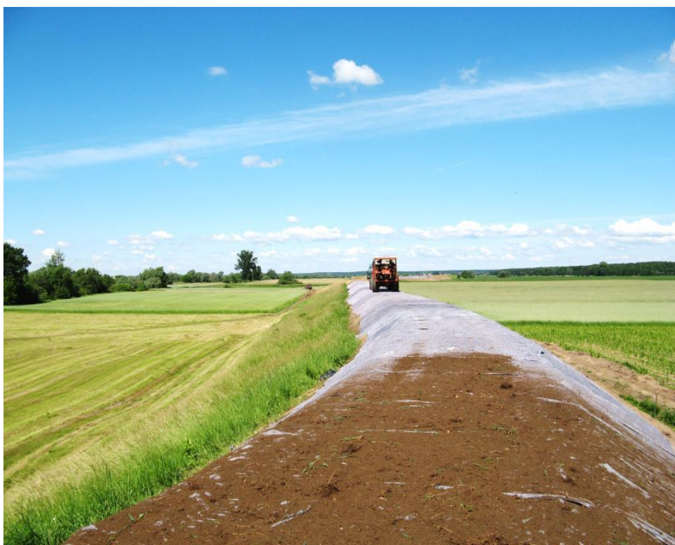
Fot 2. Zmodernizowany wał przeciwpowodziowy w gminie Zławieś Wielka, źródło KPZMiUW
