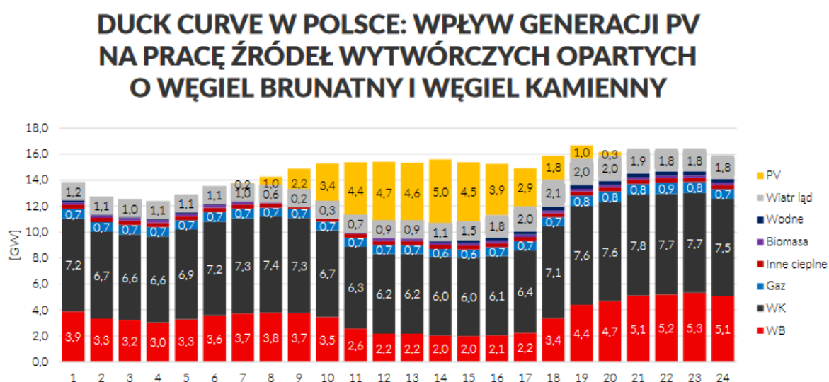
Rysunek 16. Zjawisko "krzywej kaczki" (źródło: Instytut Jagielloński)
