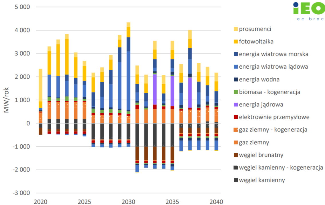
Rysunek 11. Bilans wyłączeń i nowych mocy wprowadzanych do krajowego systemu elektroenergetycznego (źródło: Instytut Energetyki Odnawialnej)
