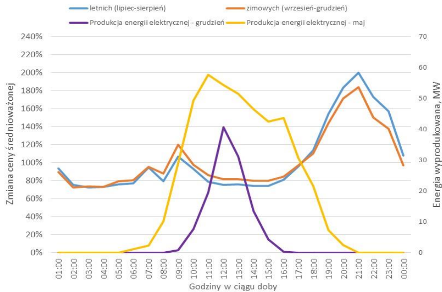
Rysunek 17. Wpływ krzywej kaczej na cenę energii w profilu dobowym (źródło: opracowanie własne)
