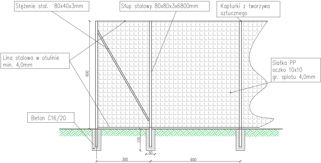
Schemat piłkochwyty skala 1:100
